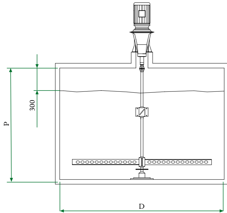
Schema vasca in cemento per agitatore tipo: S20 - S30 - S40 - S50
