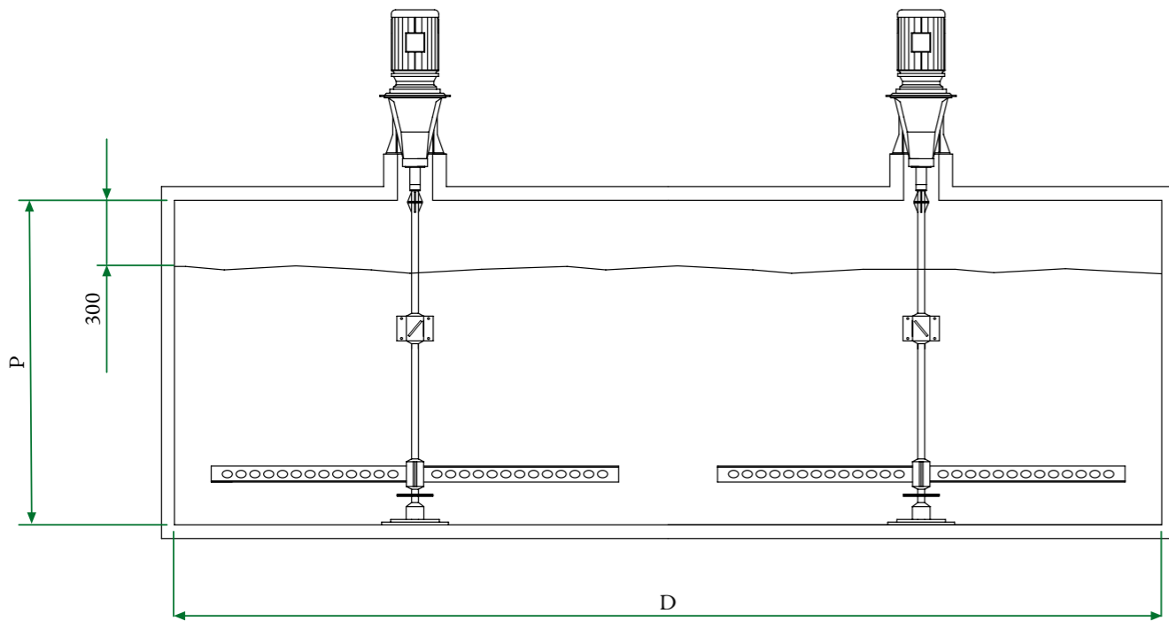
Schema vasca in cemento per agitatore tipo: S90 - S100
